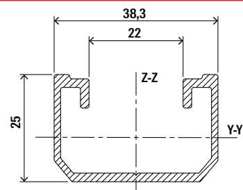
SolarMetal L H25 AL
