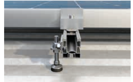
Toiture avec couverture en tôle ondulée
