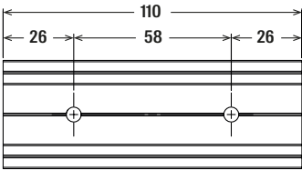
SolarMetal L 110 mm
