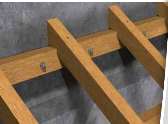
Fixation d'une muraillière sur béton
